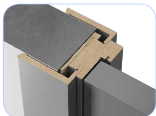
Короб телескоп, наличник Прямой
