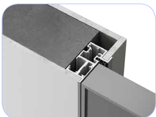
Короб INVISIBLE ALU / INFINITY
