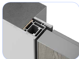
Короб Invisible 60U, прямое открывание
