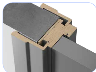
Короб телескоп, наличник Тип 2
