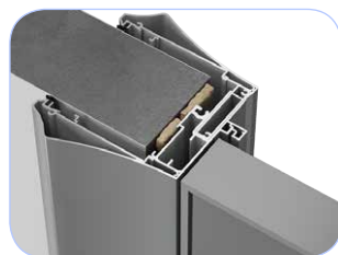
Короб INTEGRAL, наличник Фигурный
