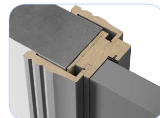
Короб телескоп, наличник Тип 4
