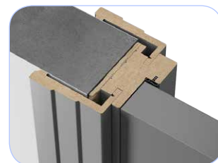
Короб телескоп, наличник Тип 3
