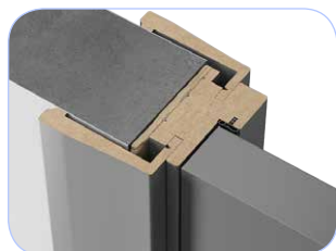
Короб телескоп, наличник Тип 1
